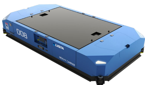
LISTA Heavy Carrier per il trasporto di grossi pesi da 3 a 8 t
